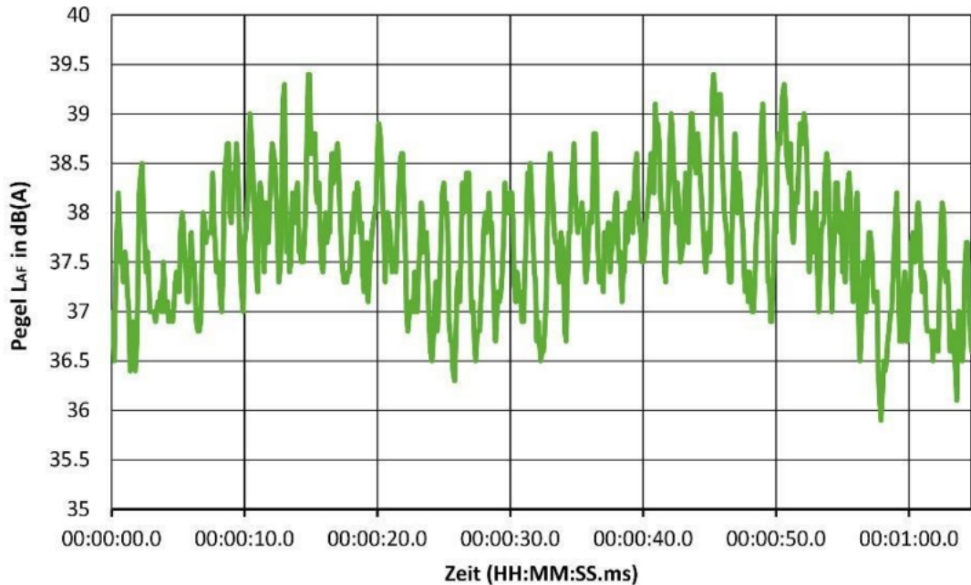
Abbildung 3: Exemplarischer Pegelschrieb bei vorliegender Amplitudenmodulation
